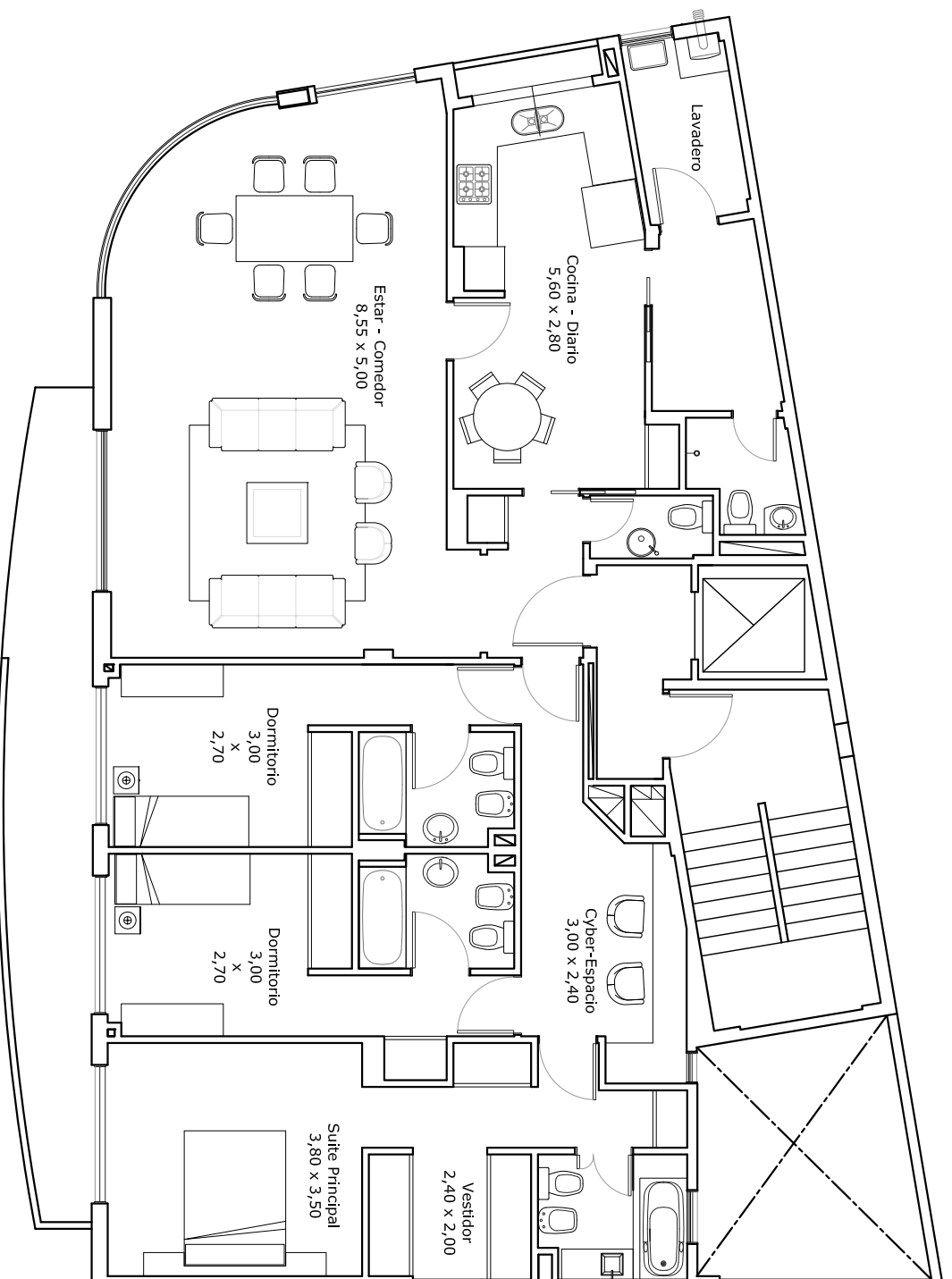
Planta Tipo 2º al 8º
