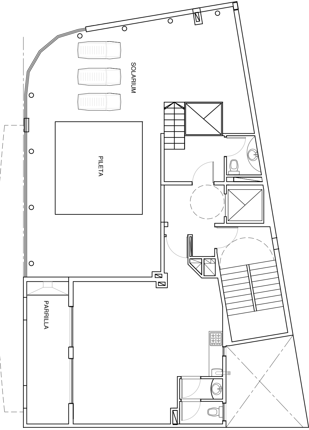
Planta 9° piso Pileta - Parrilla
